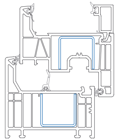
Elegante profilé non recouvert · Échelle 1:2
