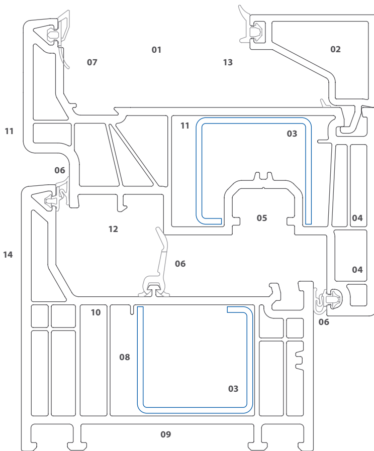
Elegante profilé recouvert Échelle 1:1
