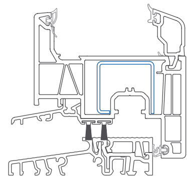
Elegante avec un seuil chaud en aluminium et une baguette arrondie · Échelle 1: 2
